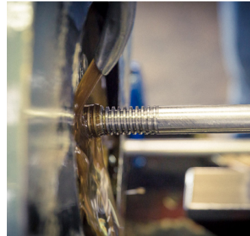
MACHINE À FILETER HOTTIAUX et WAGNER Ø6 à 50 Pas métrique, trapézoïdal, Sellers, whitworth, rond
