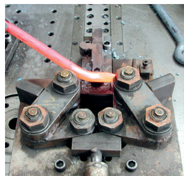
PRESSES HORIZONTALES HYDROIL de 10 à 35 t Cintrage maxi 50 mm
